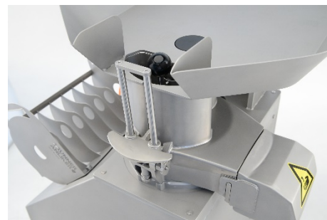
Abb. 38: Stössel unten
