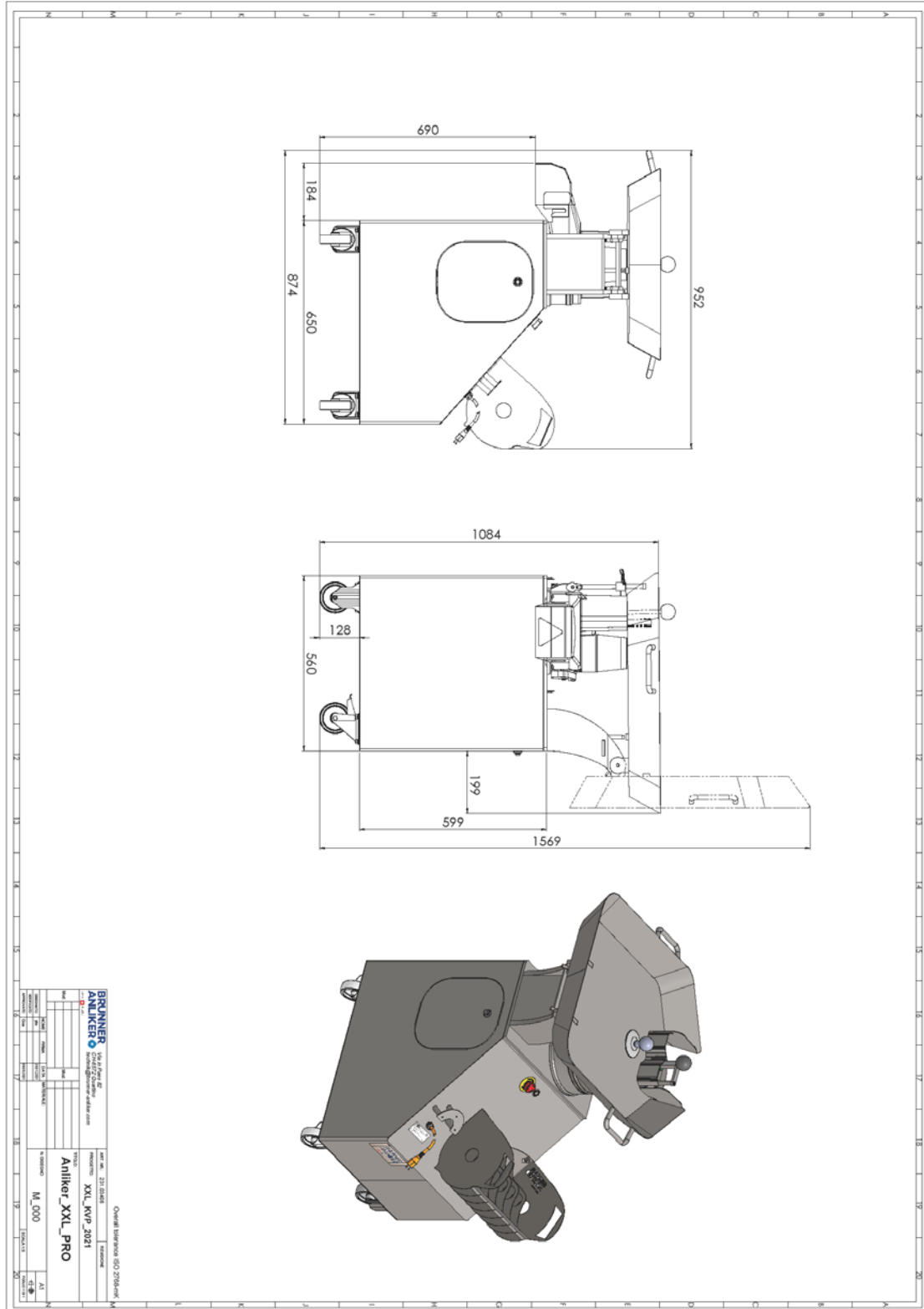
Abb. 45: Massbild ANLIKER XXL PRO
